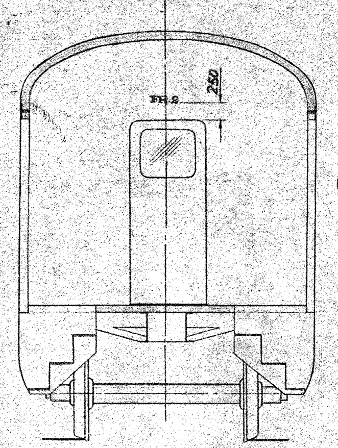
Corte B-B
