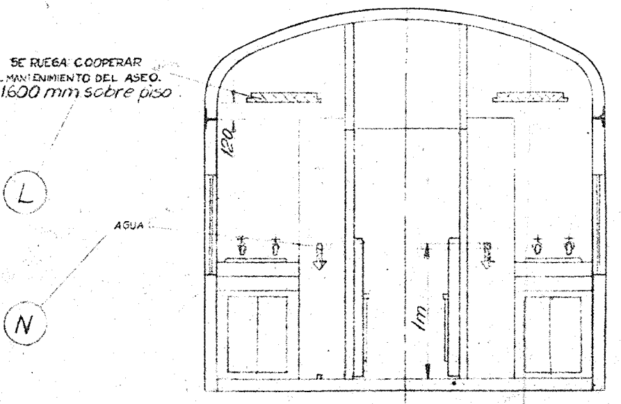
Corte C-C
